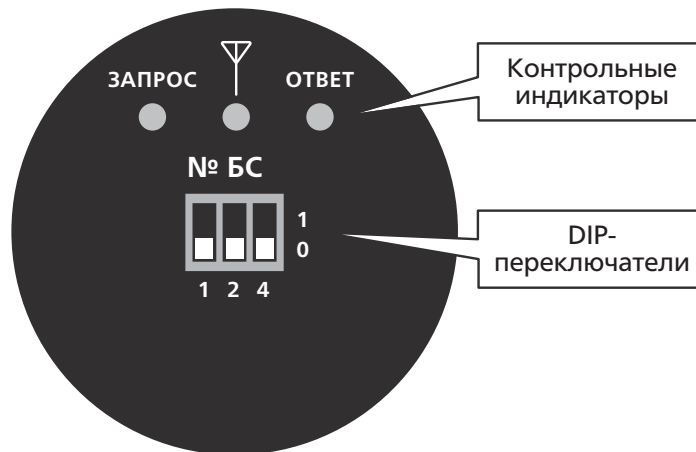
РИСУНОК 1.5. Табло БИВ3 – ISM868/RS485.
