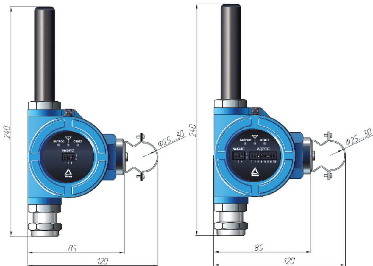
РИСУНОК 1.7. Габаритно-монтажные размеры БИВЗ – ISM868/RS485 и БИВ2-UART/ISM868
