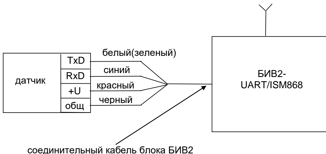
Рисунок 1.2 - Схема подключения БИВ2-UART/ISM868 к первичному преобразователю (датчику).
